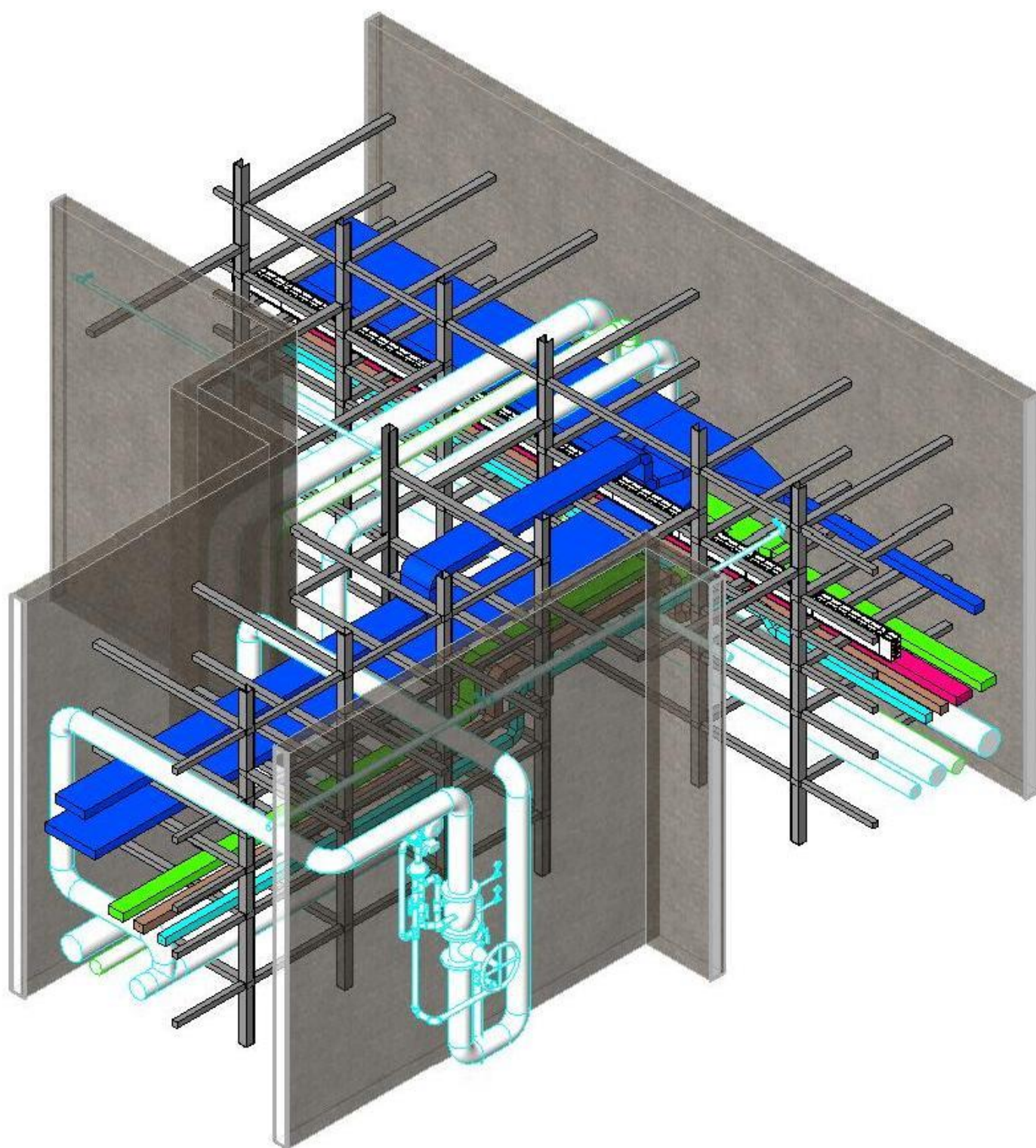
Galeria Técnica - Shopping Pelotas-RS Perspectiva das instalações em Revit MEP
